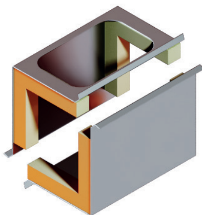
Обечайка для установки на ребро
