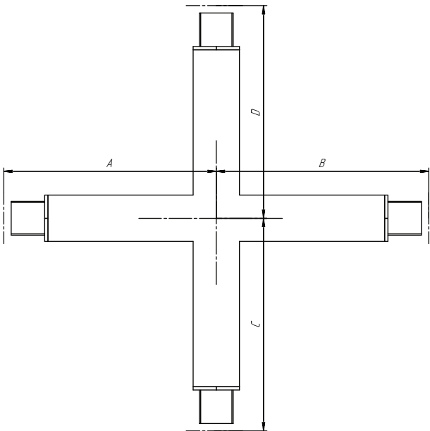
Крестовина вертикальная
